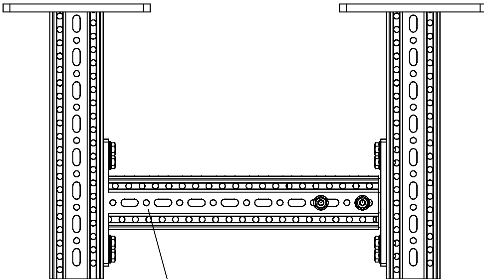
Standard- Auslegerkonsole AK F 80 + Stirnadapter STA F 80
